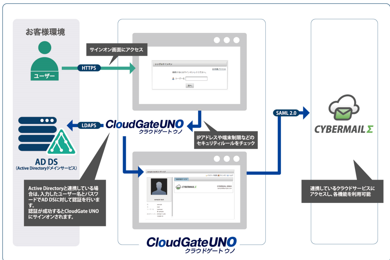
CYBERMAILΣとCloudGate UNO のログインシーケンス図
